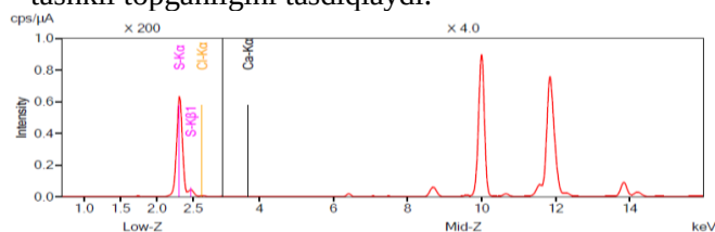
1-rasm. Sulfolangan polivinilxlorid (PVX-SO 3 Ca) ED-XRF spektri
